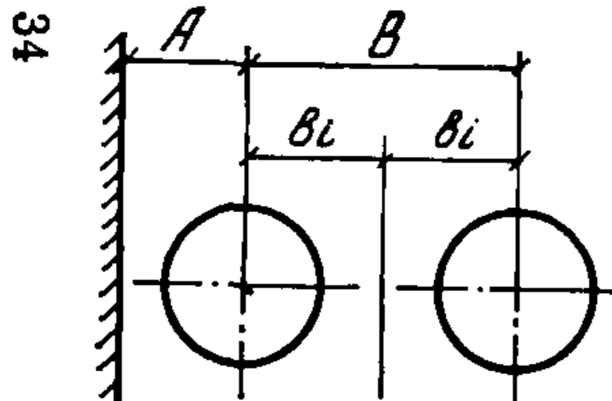
Расстояния между осями смежных трубопроводов и от трубопроводов до стенок каналов, тоннелей, галерей и стен зданий, мм
